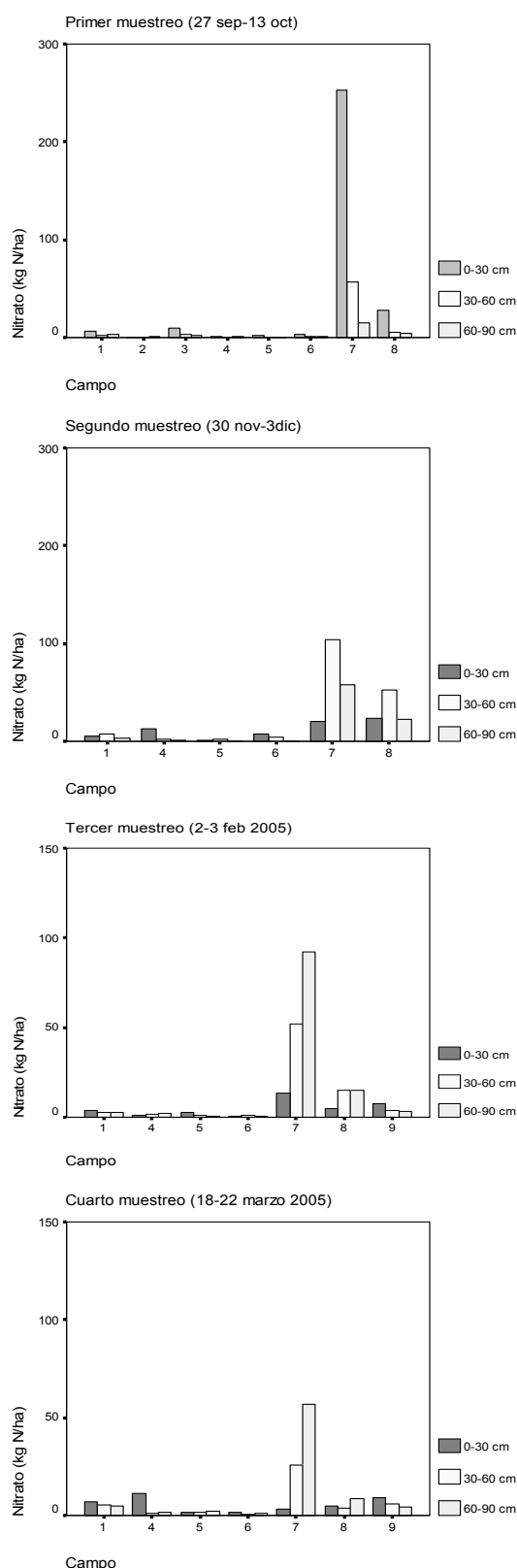
Fig. 2. Contenidos de nitratos por profundidades en los diferentes muestreos.
