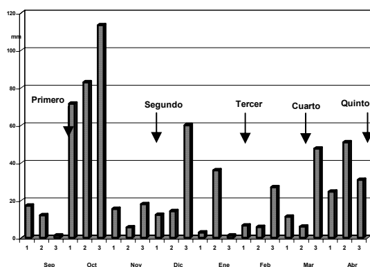
Fig. 3. Pluviometría acumulada entre muestreos.
