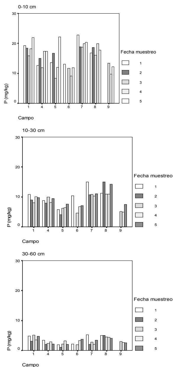
Fig. 4. Concentraciones de P Olsen en las profundidades de 0-10, 10-30 y 30-60 cm en los cinco muestreos de suelo llevados a cabo.
