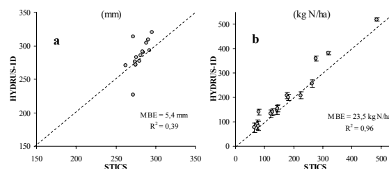
Fig. 5. Correlación de los valores simulados finales (18/06) de drenaje acumulado (a) y lixiviación (b) con los códigos STICS e HYDRUS-1D por debajo de los 1,2 m de profundidad del suelo.
