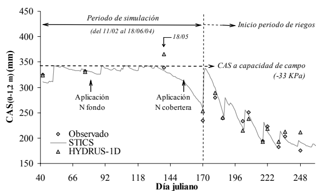
Fig. 1. Contenido de agua al suelo (CAS) en los primeros 1,2 m de profundidad del suelo del tratamiento N2T2 repetición 2 del ensayo. Valores observados y simulados con STICS e HYDRUS-1D durante toda la campaña del maíz el año 2004.
