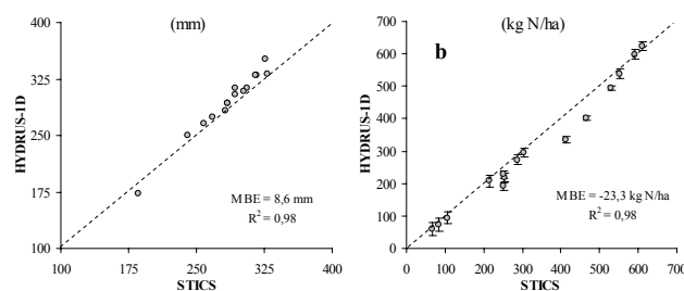
Fig. 3. Correlación de los valores simulados finales (18/06) de CAS (a) y de CNS (b) con los códigos STICS e HYDRUS-1D de los primeros 1,2 m del perfil del suelo.
