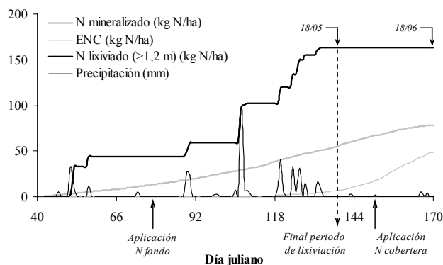
Fig. 2. Contenidos de nitrógeno mineralizado, extracciones de nitrógeno del cultivo (ENC), nitrógeno lixiviado y precipitación caída en los 1,2 m de perfil superficial del suelo. Valores simulados con el código STICS en el tratamiento experimental N2T1 repetición 2 del ensayo.
