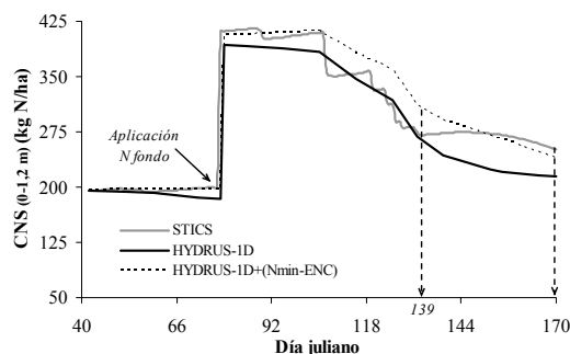
Fig. 4. Evolución de los CNS simulados con STICS, HYDRUS-1D e HYDRUS-1D más la diferencia entre el nitrógeno mineralizado (Nmin) y las extracciones de nitrógeno del cultivo (ENC) simulados por STICS. Valores del tratamiento NIT2 repetición 3 del ensayo.
