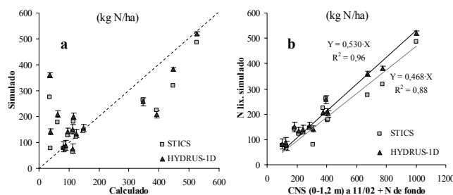
Fig. 6. Estimación de los riesgos de lixiviación de nitratos simulados con STICS e HYDRUS-1D respecto a (a) los valores calculados por balance de nitrógeno y (b) a los CNS potencialmente lixiviables de los escenarios evaluados.
