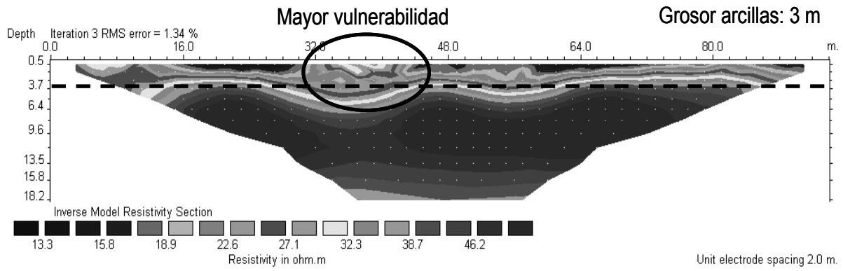
Fig. 4. Pseudosección de resistividades aparentes obtenida después de la inversión en la depresión del Empordà. El escaso espesor de la capa de arcillas aflorante y su carácter discontinuo confieren una elevada vulnerabilidad al acuífero aluvial subyacente.
