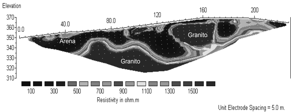
Fig. 5. Pseudosección de resistividades aparentes obtenida sobre los niveles de alteración de la granodiorita del plutón de Alforja. En el perfil se refleja claramente la irregularidad del relieve del basamento, con la presencia de bolos de elevada resistividad.
