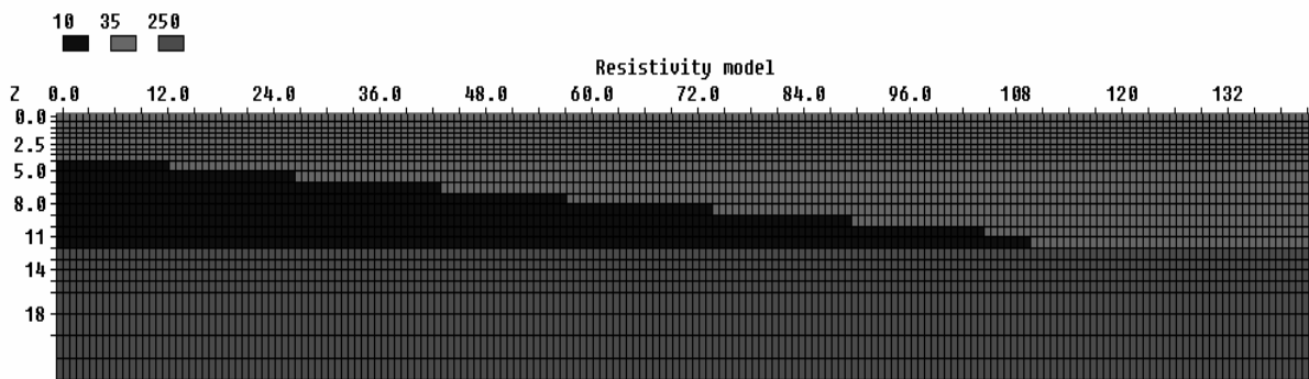
Fig. 2. Modelo sintético simulando un acuífero situado a 12 metros de profundidad, cubierto por una zona no saturada constituida por un nivel de arcillas que se acuña bajo otro nivel superior arenoso.
