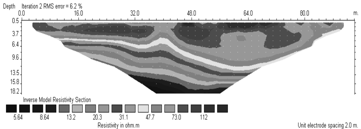
Fig. 6. Pseudosección de resistividades aparentes obtenida sobre la terraza aluvial del valle bajo del río Llobregat. La ausencia de niveles conductores en la zona no saturada implica el elevado riesgo de contaminación por vertidos contaminantes en este contexto. En cambio, la geometría del sustrato impermeable constituido por las arcillas rojas de Burdigaliense destaca claramente en la parte inferior de la sección.
