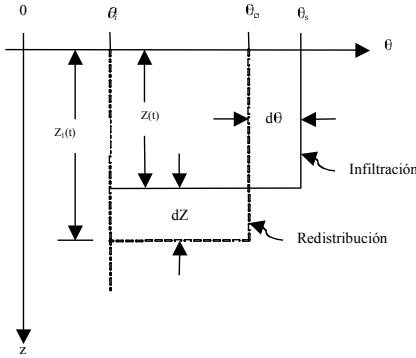
Fig. 1. Elongación del perfil de humedad durante la redistribución entre sucesos de lluvia propuesto por GAR (Ogden y Saghafian, 1997).
