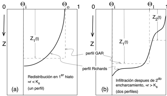
Fig. 2. Método de cálculo de redistribución de humedad usando dos perfiles superpuestos.
