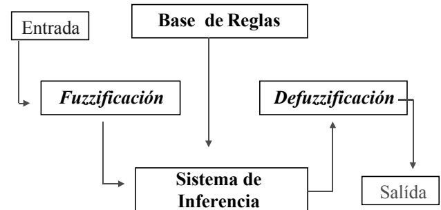
Fig.1 Configuración del modelo basado en reglas fuzzy.
