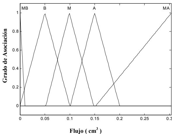
Fig.3. Conjuntos fuzzy asociados a las variables de salida “densidad de flujo”.
