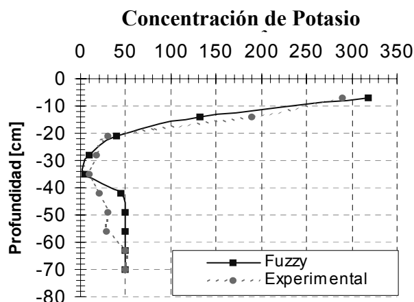
Fig.5 Concentración de potasio observada y simulada a través del MBRF.
