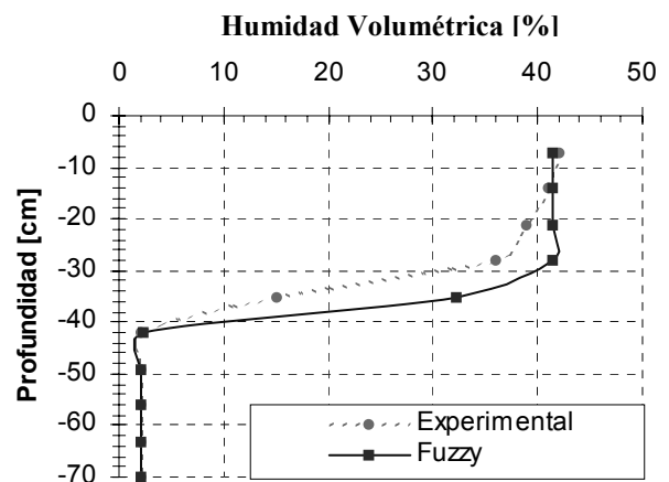
Fig.4. Humedad Volumétrica observada y simulada a través do MBRF.
