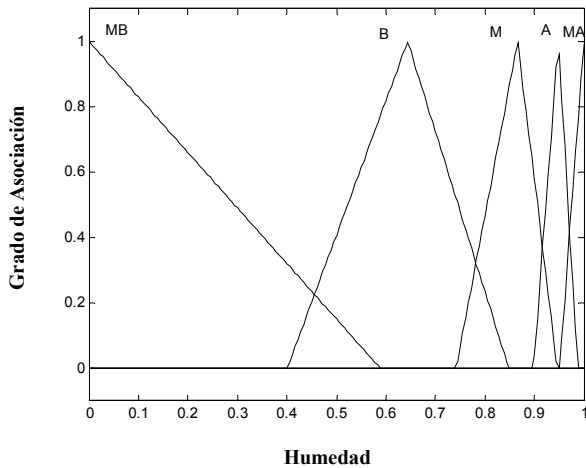
Fig.2 Conjuntos fuzzy asociados a las variables de entrada “razón de humedad”.
