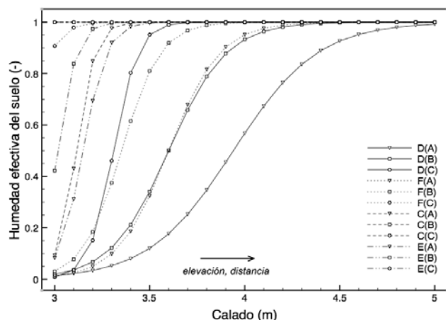
Fig. 6. Relaciones sigmoideales entre humedad efectiva del suelo y calado desarrollado para cada localización y profundidad.
