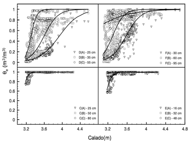
Fig. 5. Relación entre el calado del río y la humedad efectiva del suelo en la llanura de inundación a varias distancias y profundidades.
